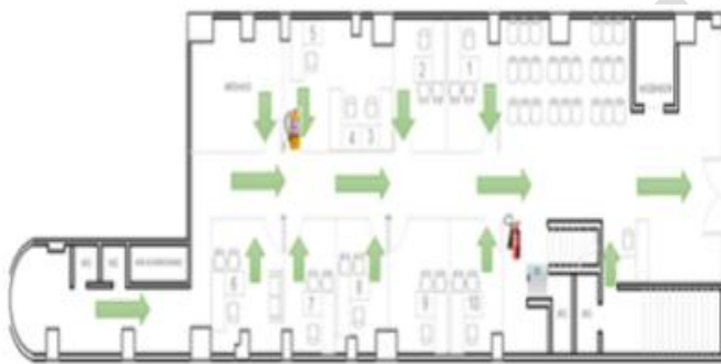
PLANTA 1er NIVEL 10 PUESTOS DE TRABAJO - ESC:125
