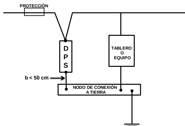
FIGURA MONTAJE TÍPICO DE DPS
